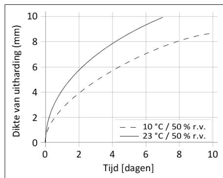
Schema 1: Uithardingsnelheid Sikaflex®-290 DC PRO
