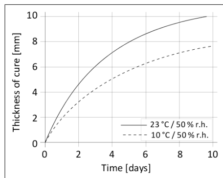
Schema 1: Uithardingsnelheid Sikaflex®-515
